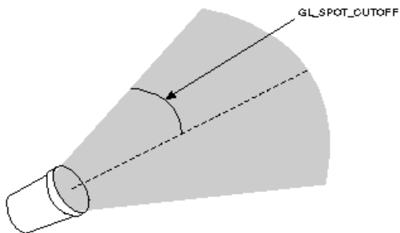
Figure 5-2 : GL_SPOT_CUTOFF Parameter
