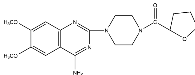
Terazosin (Hytrin)
