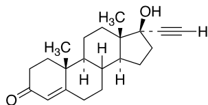
Ethisterone
