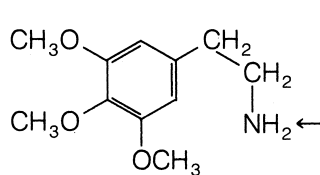
Mescaline
