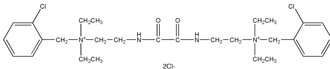
Ambenonium Chloride
