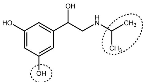
Metaproterenol
