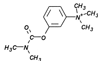
Neostigmine
