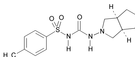
gliclazide
