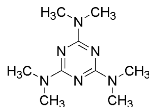
Altretamine
