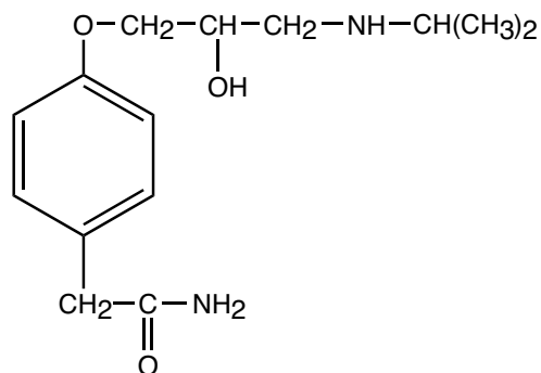
Atenolol (Tenormin)
