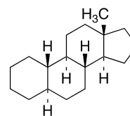
5 \alpha -Estrane
