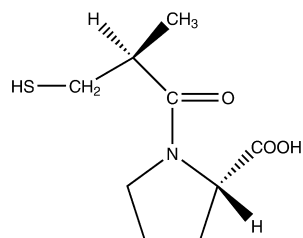
Captopril (Capoten)
