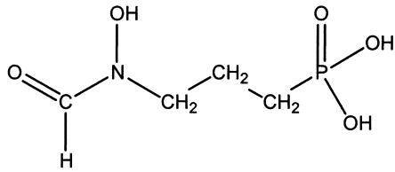
Fosmidomycin
