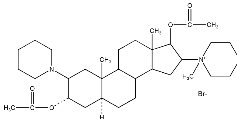
Vecoronium Bromide
