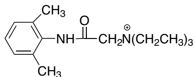
QX-314
