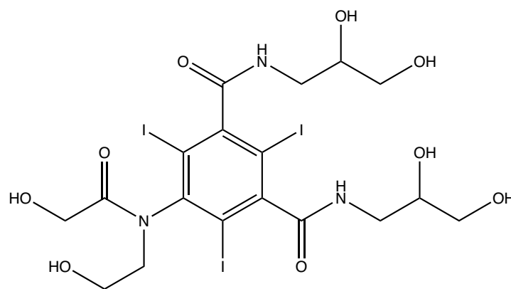
Ioversol
