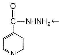
Isoniazid
